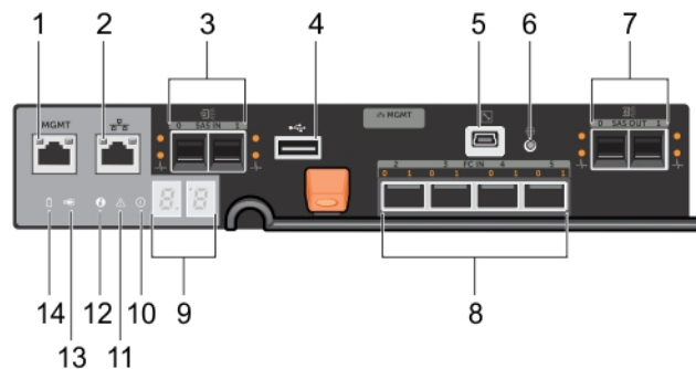
Abbildung 8. Merkmale und Anzeigen des MD3860f Fibre Channel RAID-Controller-Moduls
