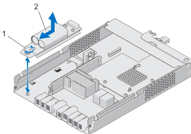
Abbildung 25. Entfernen und Installieren des RAID-Controller-Modul-Akkusicherungsmoduls
