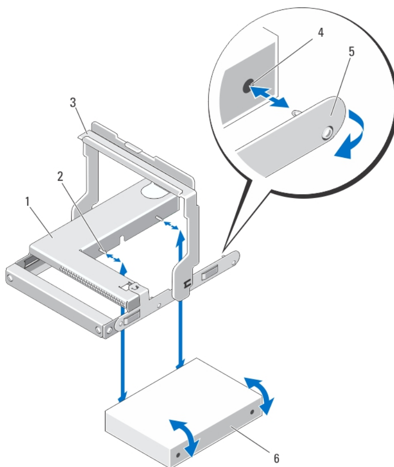
Abbildung 17. Entfernen und Installieren des physischen 2,5-Zoll- Laufwerks in einem physischen 2,5-Zoll-Laufwerksträger
