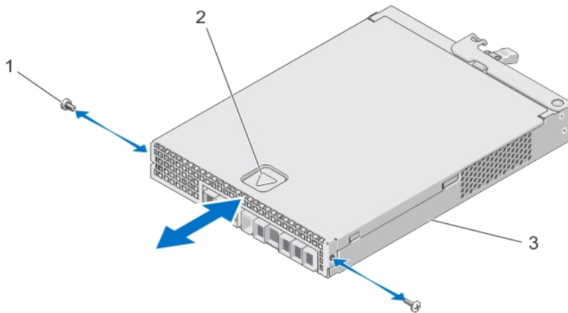
Abbildung 23. Öffnen und Schließen des RAID-Controller-Moduls
