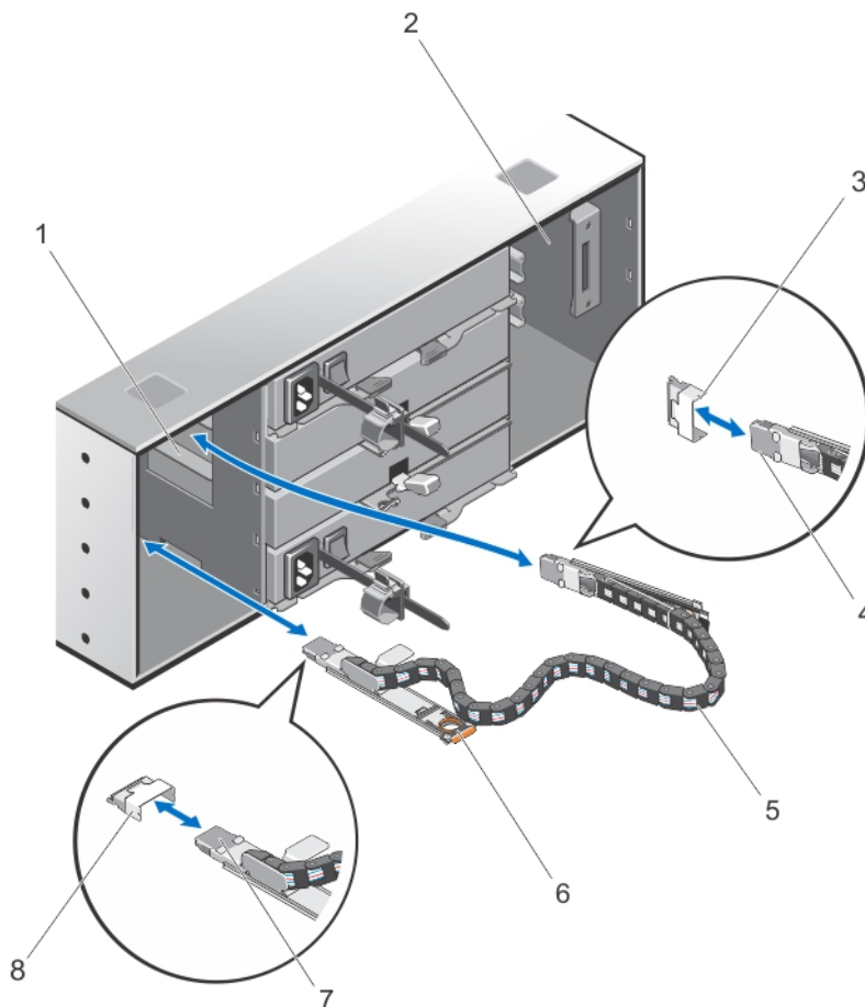
Abbildung 21. Entfernen und Installieren der/des SAS-Kettenkabel(s)
