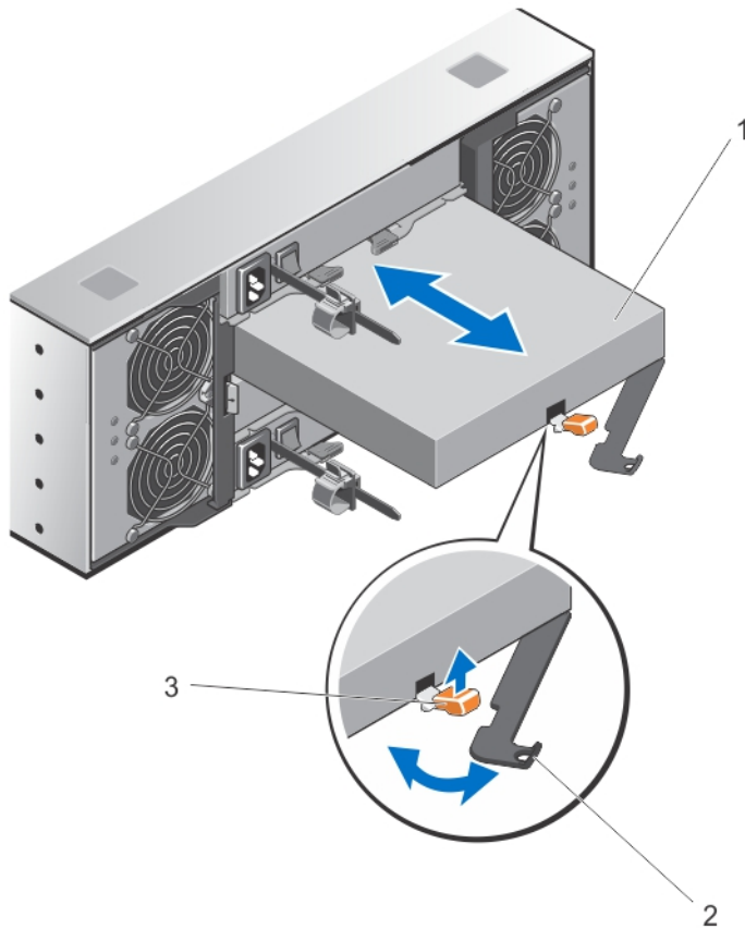
Abbildung 22. Entfernen und Installieren eines RAID-Controller-Moduls oder eines Erweiterungsmoduls
