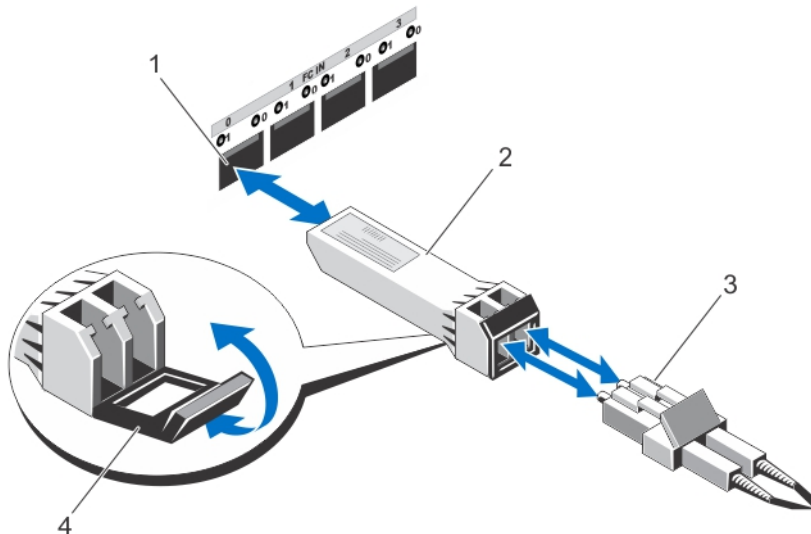
Abbildung 24. Ersetzen des SFP+-Transceivers
