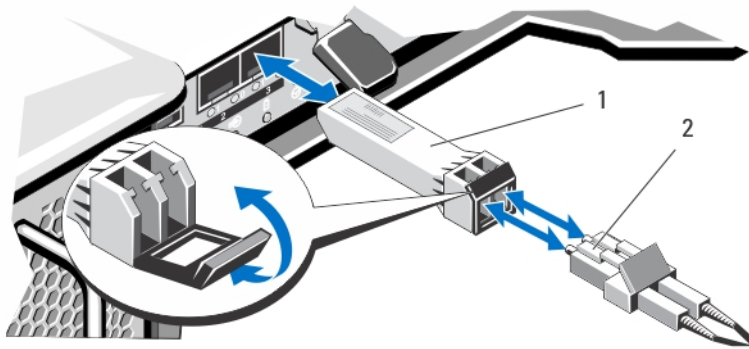
Abbildung 28. Entfernen eines SFP+-Moduls
