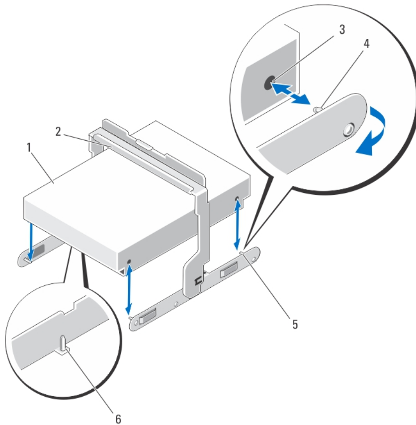
Abbildung 18. Entfernen und Installieren des physischen 3,5-Zoll-Laufwerks in einem physischen 3,5-Zoll-Laufwerksträger
