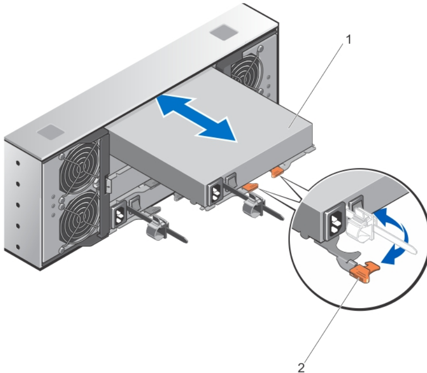
Abbildung 26. Stromversorgungsmodul entfernen und installieren
