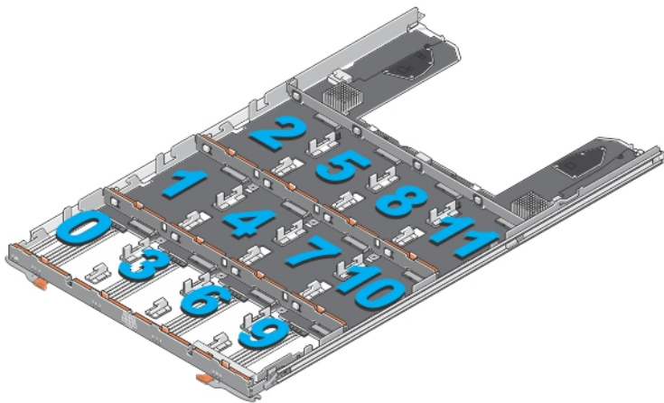
Abbildung 16. Steckplatznummerierung in der Laufwerksschublade
