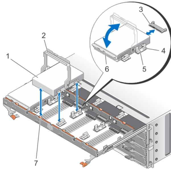
Abbildung 19. Entfernen und Installieren des physischen Laufwerks in die physische Laufwerksschublade
