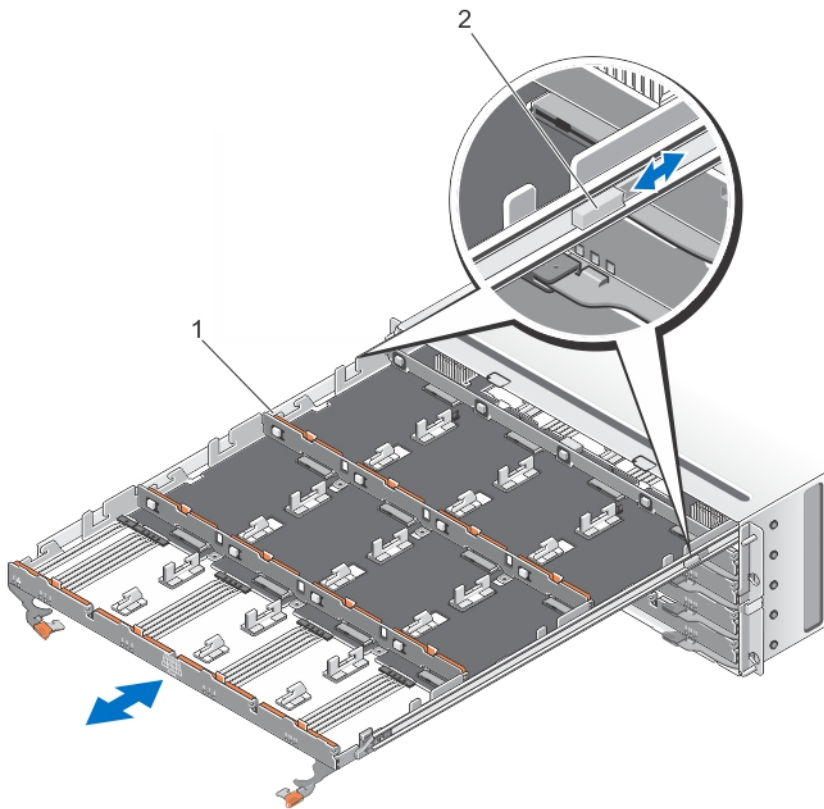
Abbildung 15. Entfernen und Installieren der physischen Laufwerksschublade
