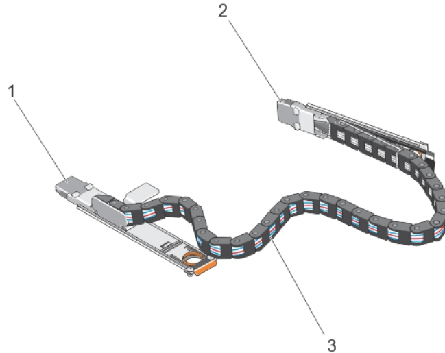
Abbildung 20. Merkmale von SAS-Kettenkabeln
