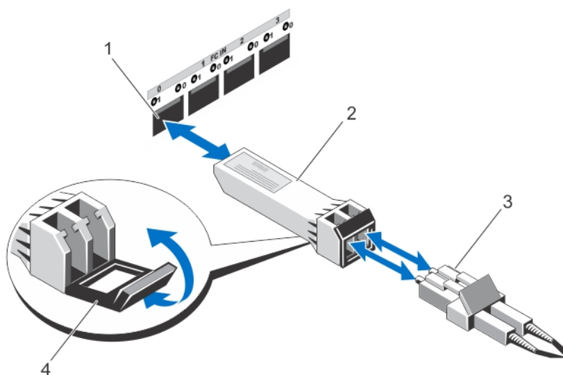
Abbildung 9. Glasfaserkabelverbindung
