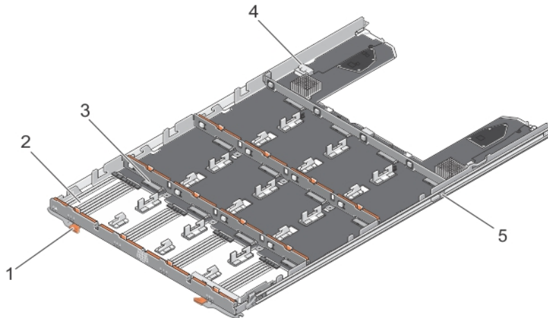
Abbildung 13. In der physischen Laufwerksschublade
