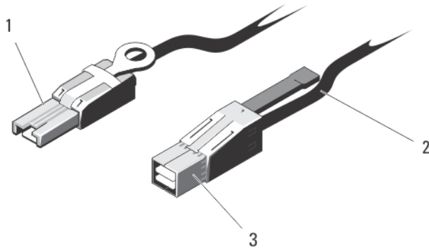
Abbildung 10. SAS-Kabel
